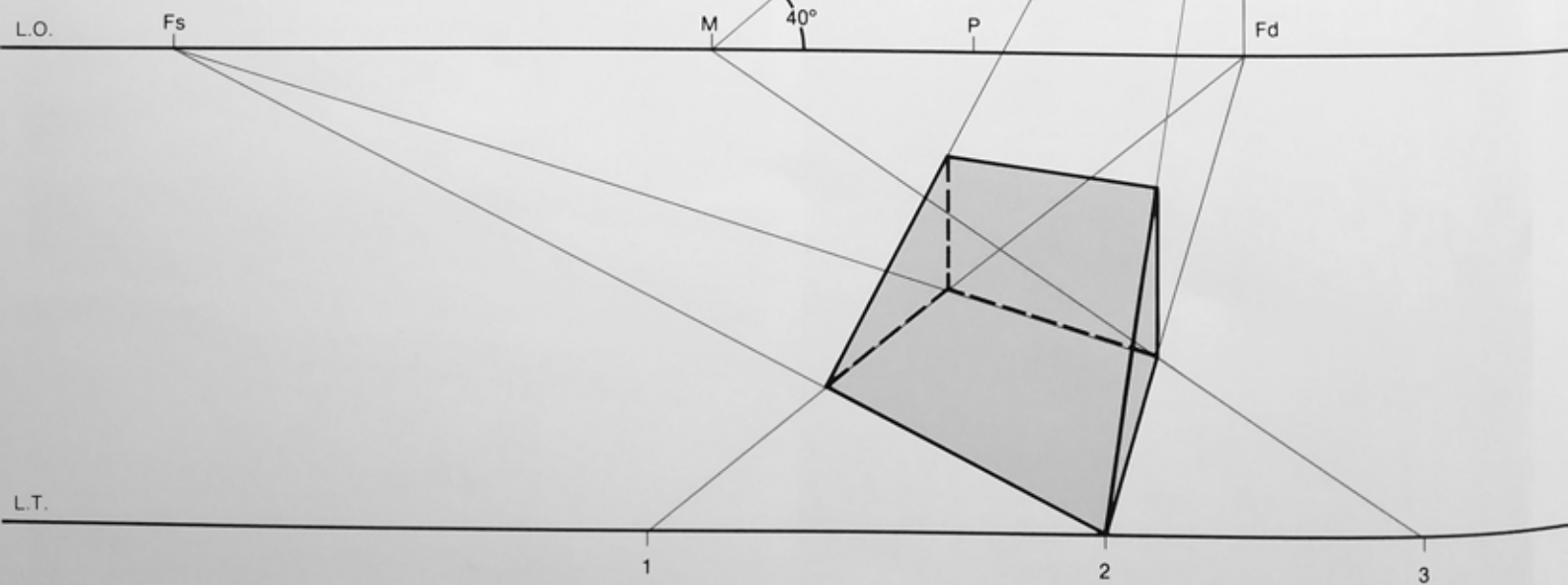
Prospettiva di un piano inclinato di 40°
