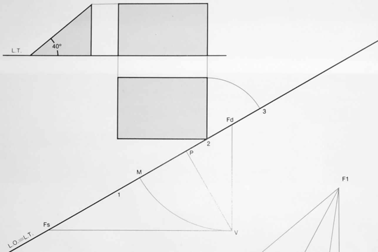
Prospettiva di un piano inclinato di 40°
