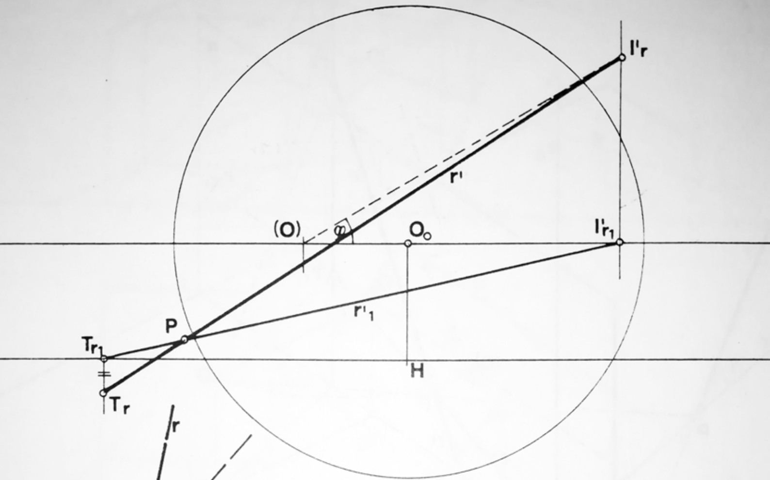
Prospettiva di una retta generica
