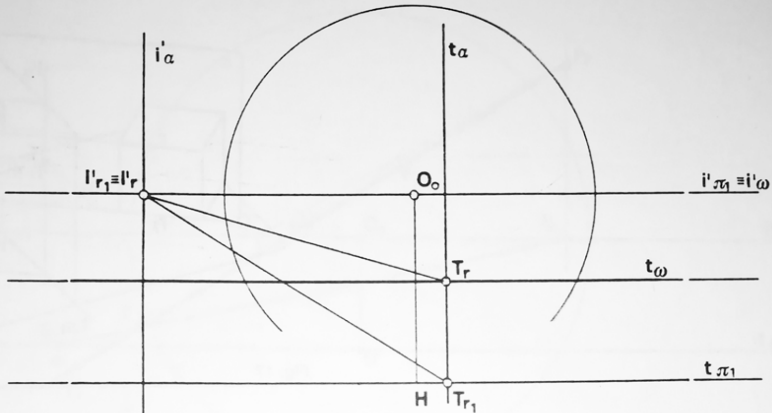
Prospettiva di una retta obliqua posta sul geometricale
