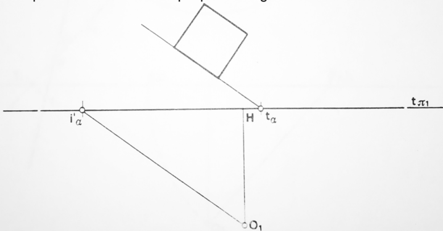
Prospettiva di una retta obliqua posta sul geometricale
